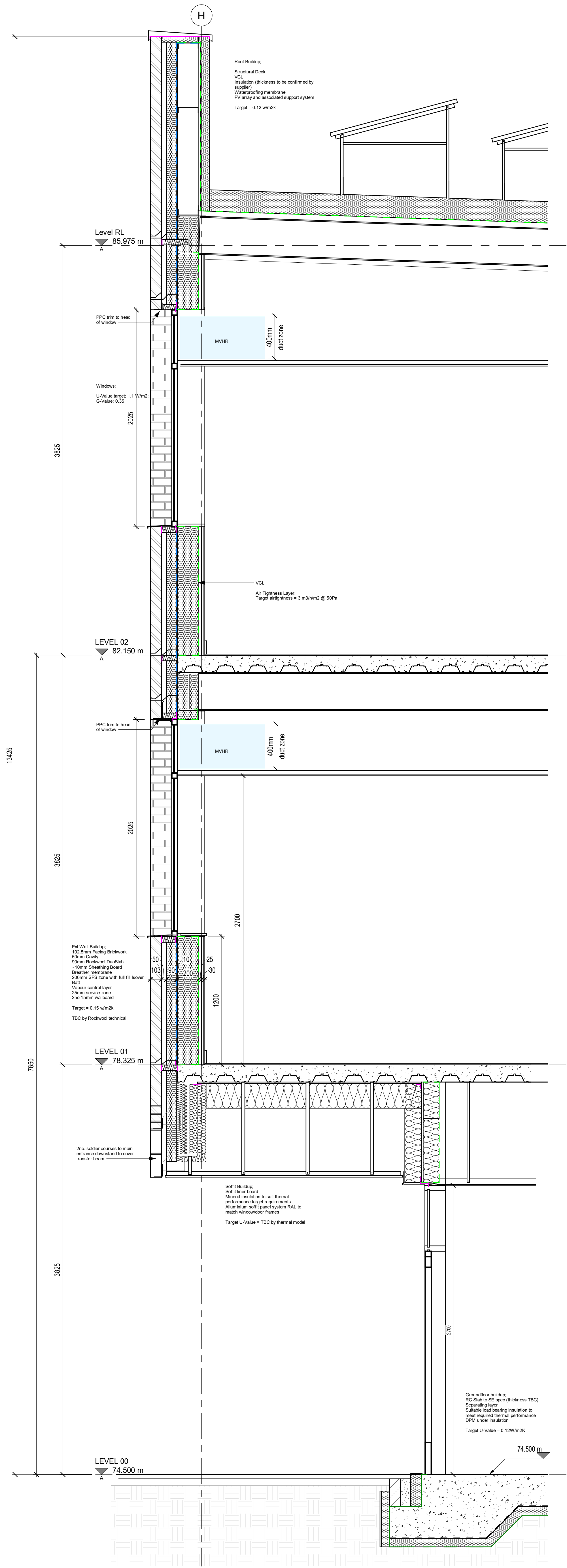
1.1 Section 1.1 1 : 20
