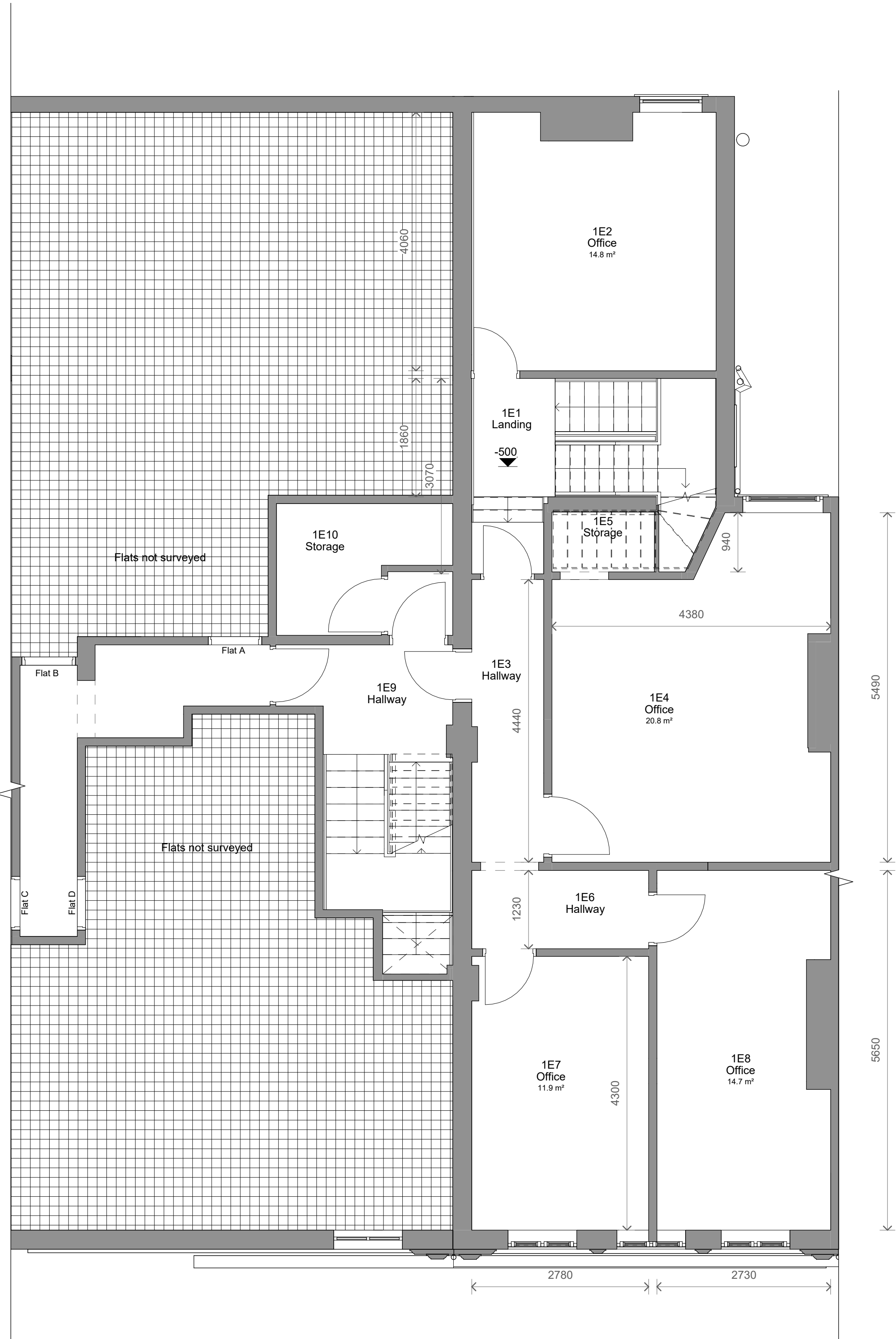
1 Level 1 - Existing 1 : 50
