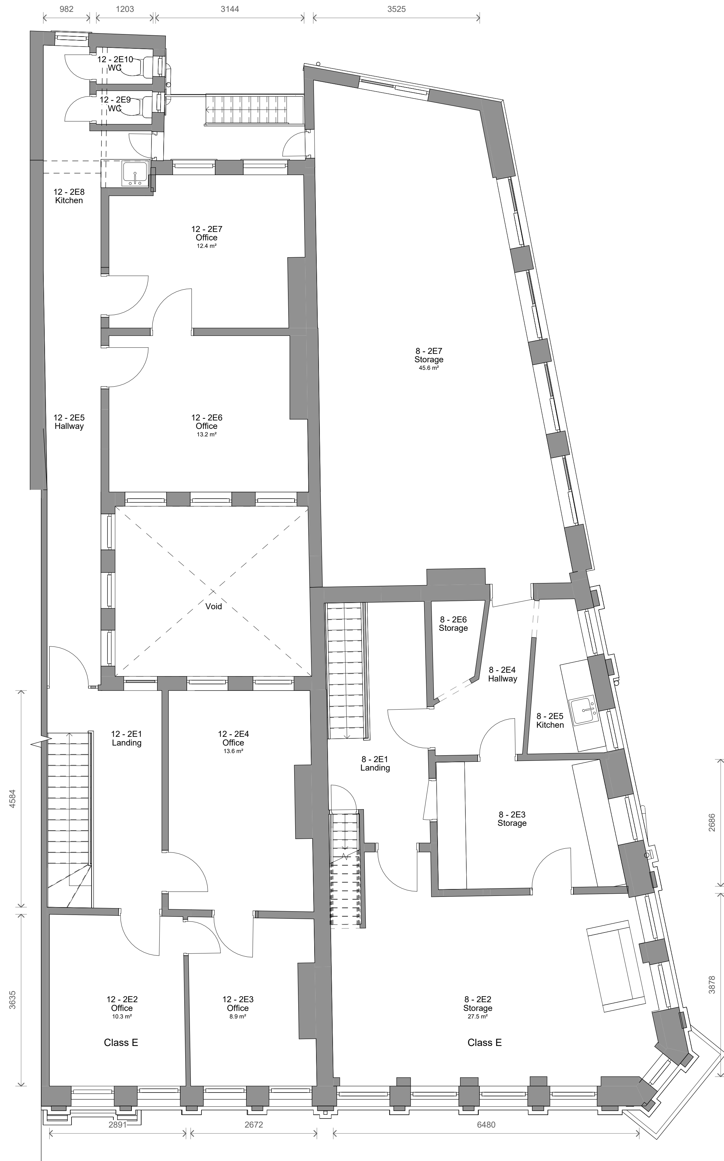
1 Level 2 - Existing 1 : 50
