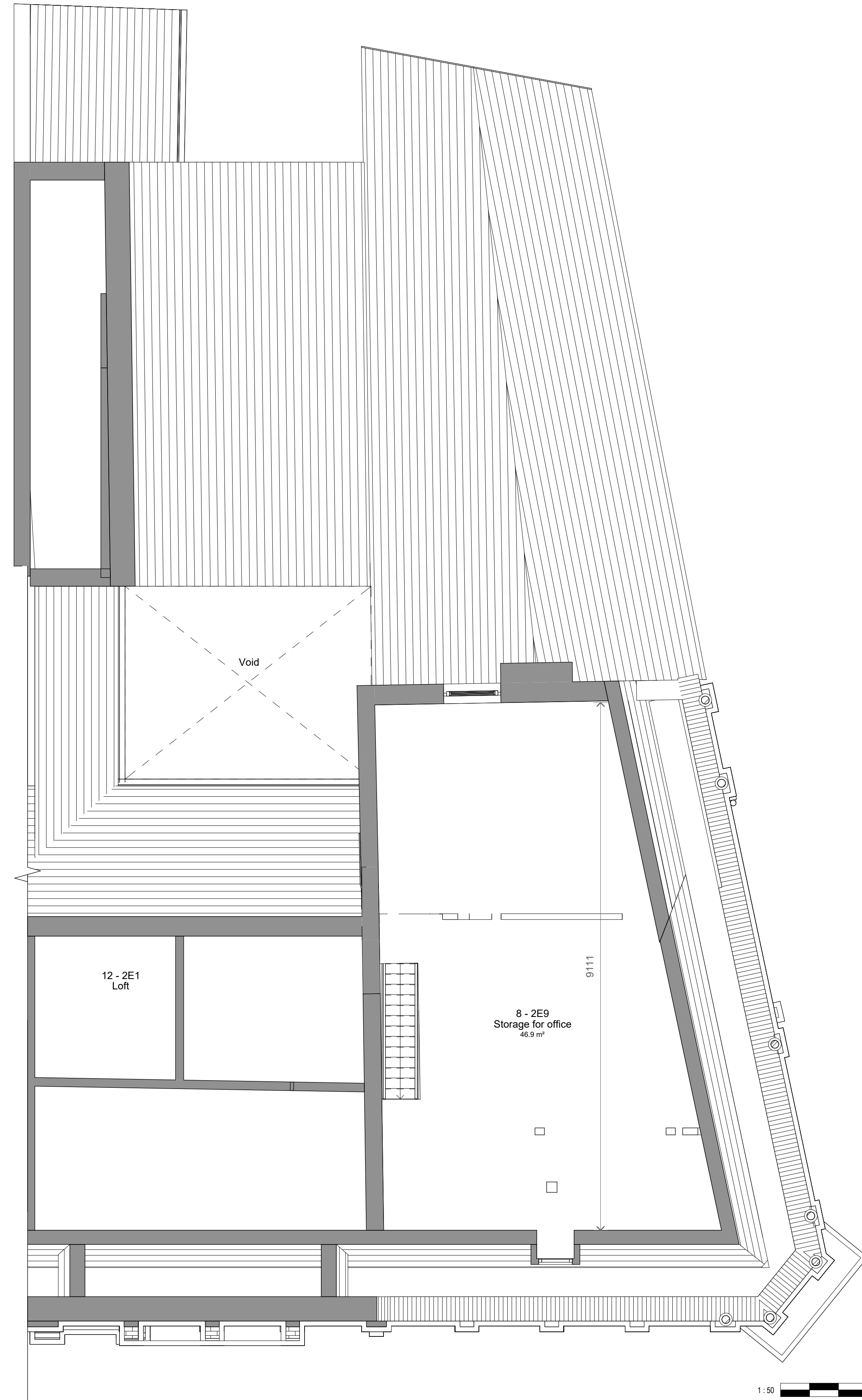
2 LEVEL 3 - Existing 1 : 50
