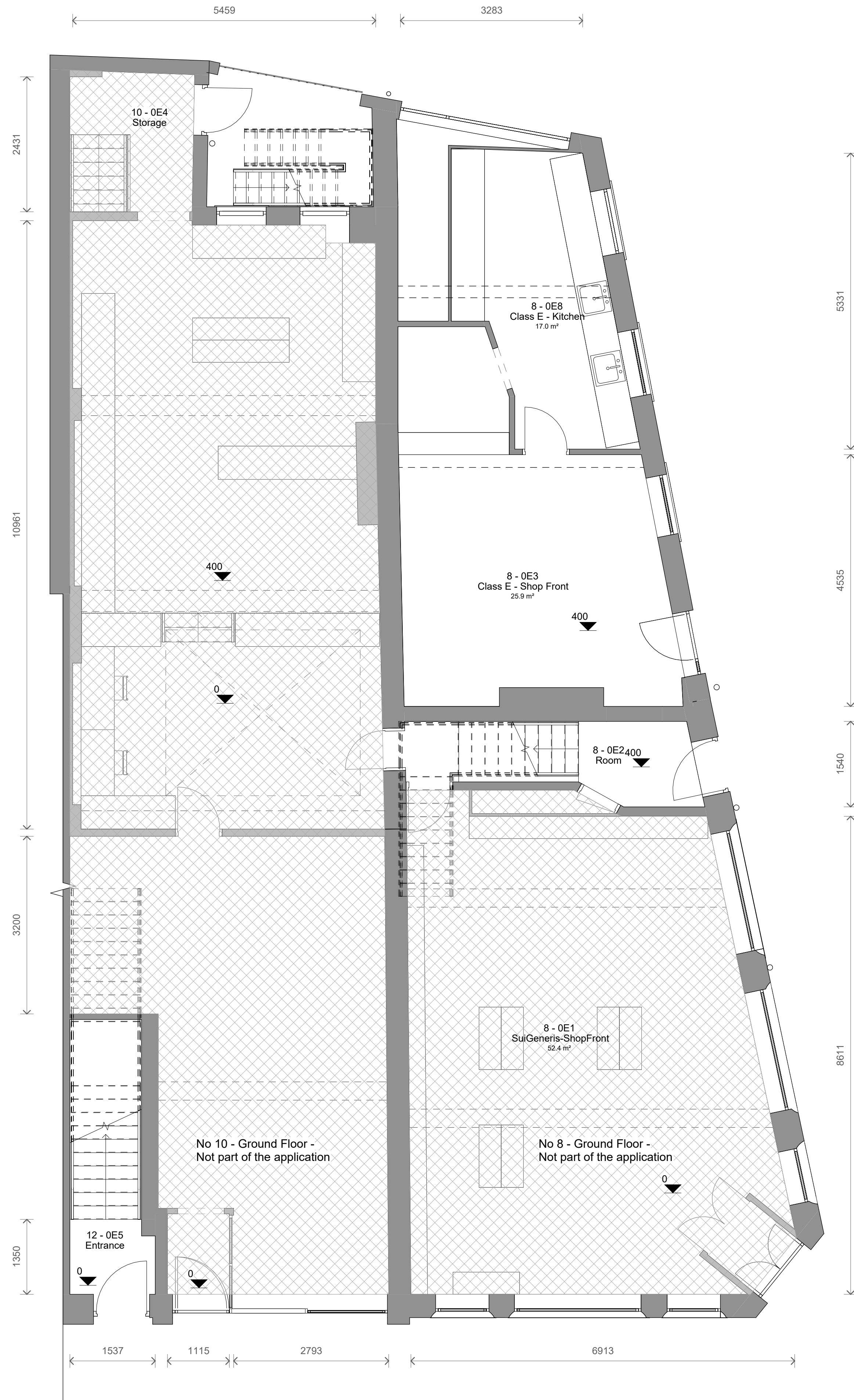
1 Level 0 - Existing 1 : 50
