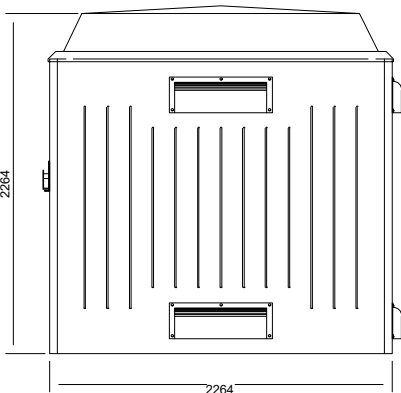
Elevation (D) (r/h side)
