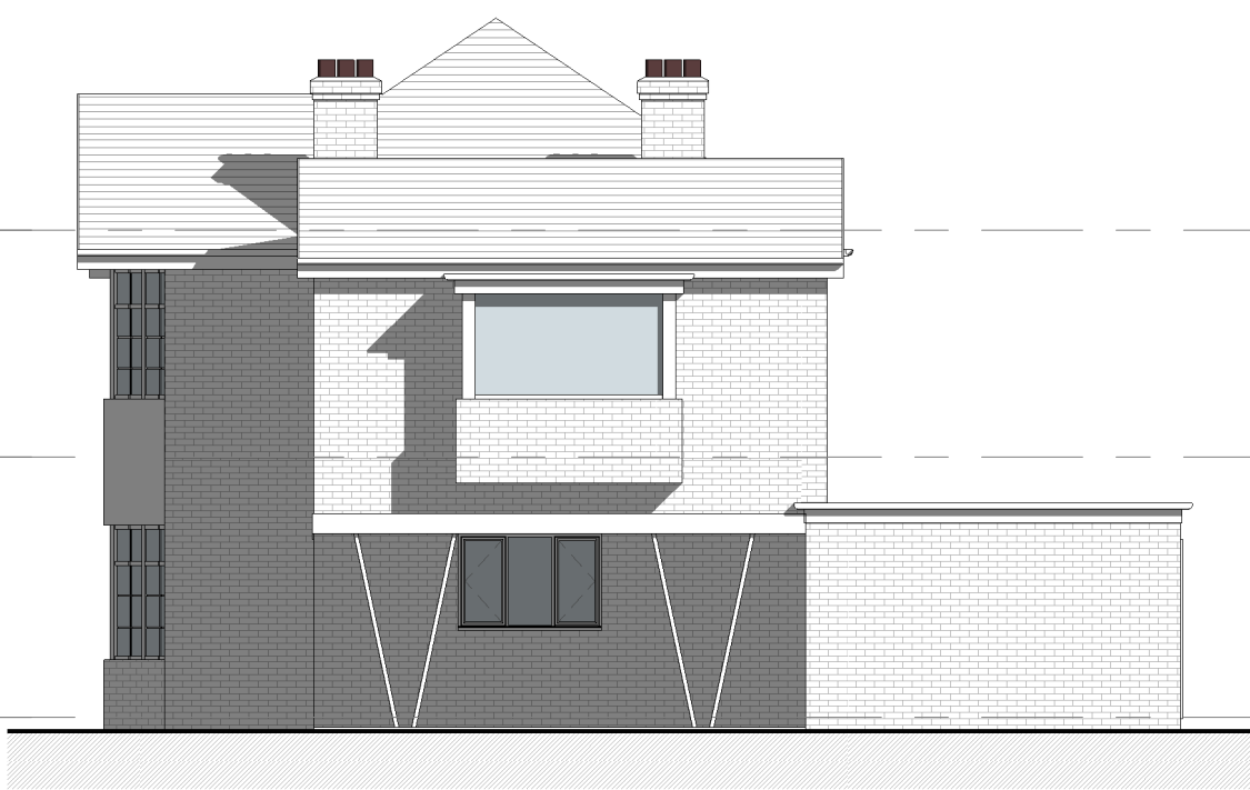
4. Right Side - Existing 1 : 100
