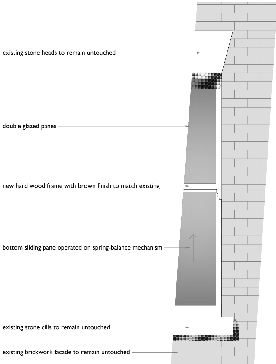
elevation
