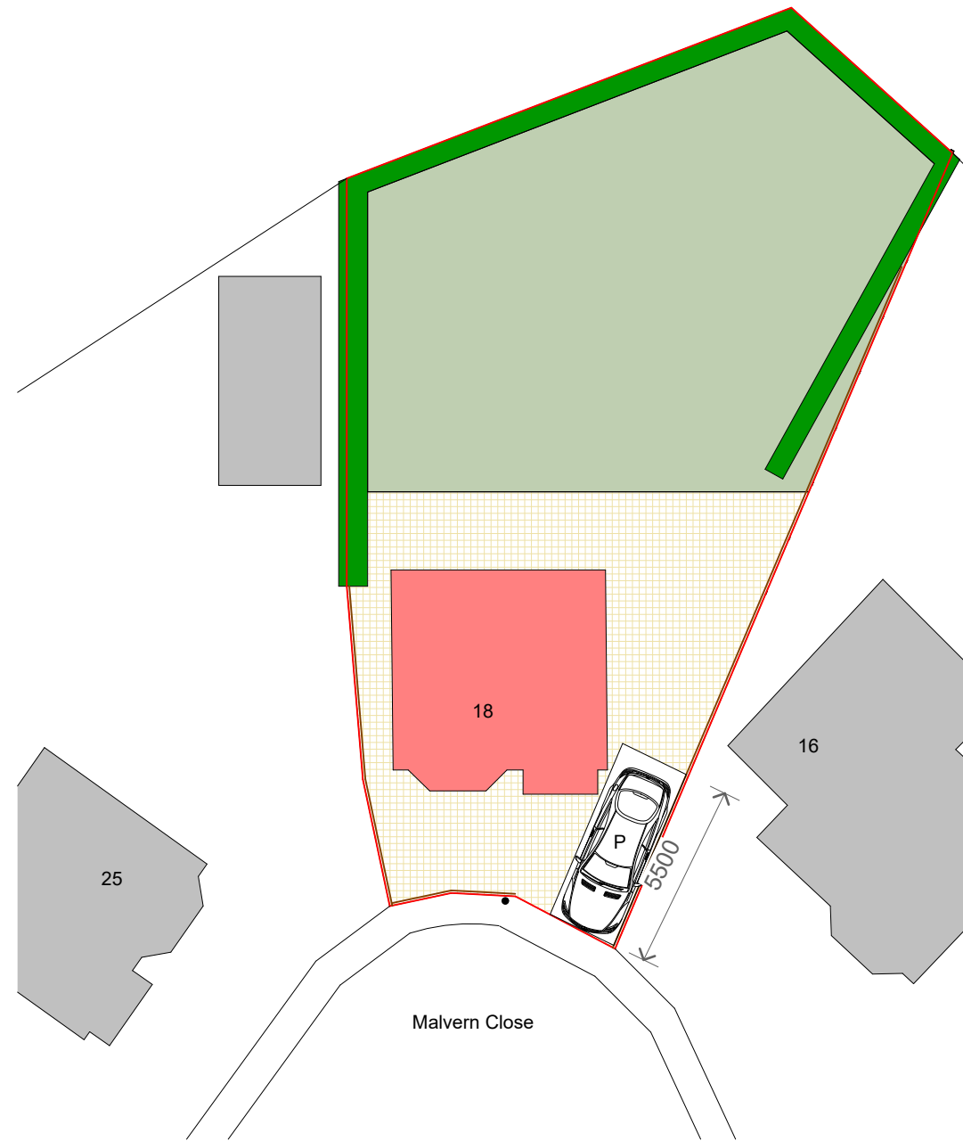
1 Site - Existing 1 : 200
