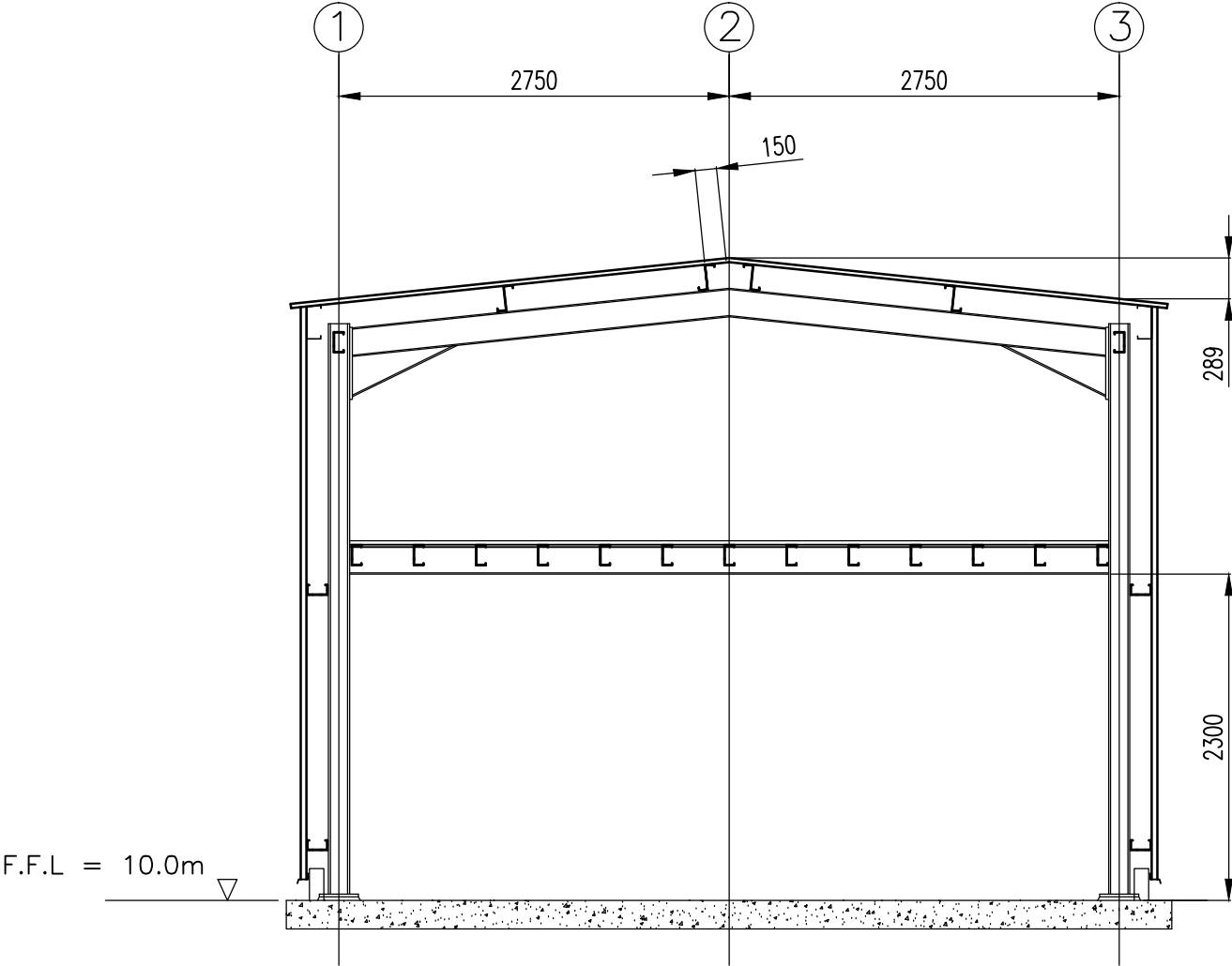
SECTION A-A 1:50
