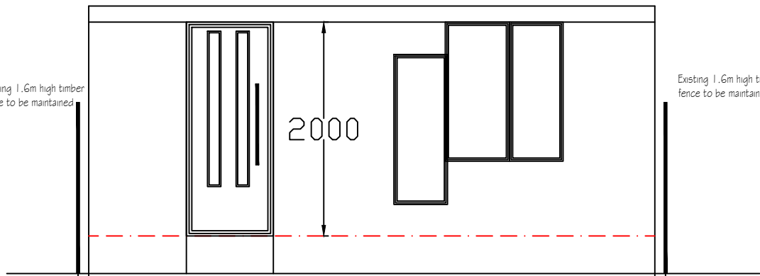
Elevation B
