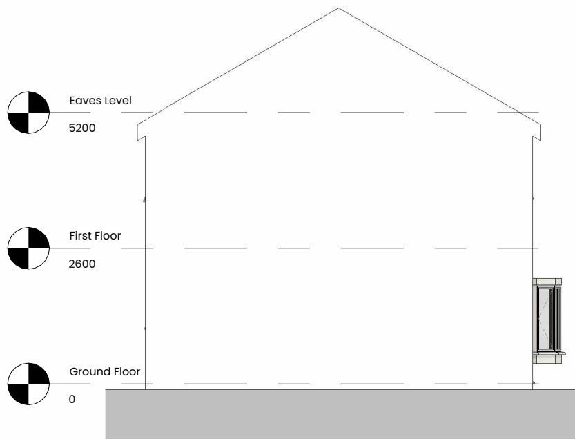
3 Existing Adjoining Elevation 1 : 100
