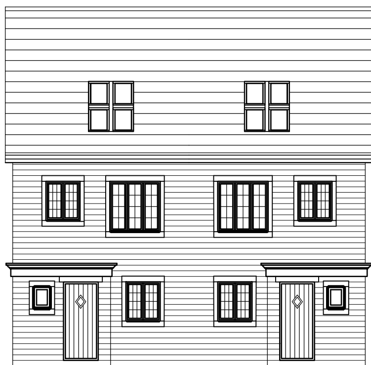
PLOTS 10 & 11 FFL-127.25
