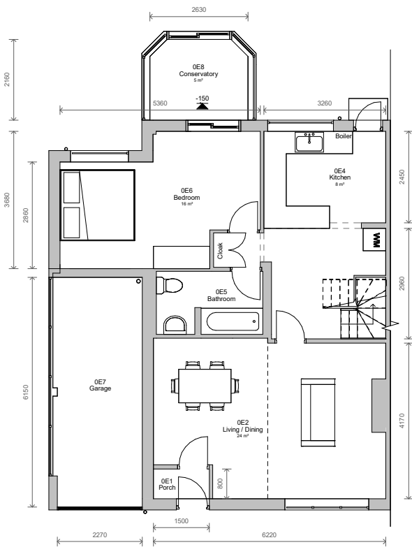
① Level 0 - Existing 1 : 50
