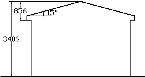
Elevation A
