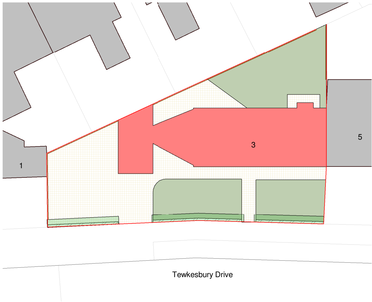
1 Site - Existing 1 : 200
