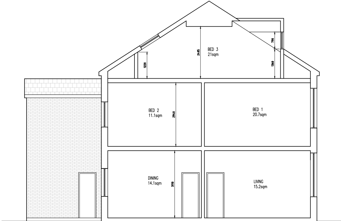
EXISTING SECTION 1:100 @ A3
