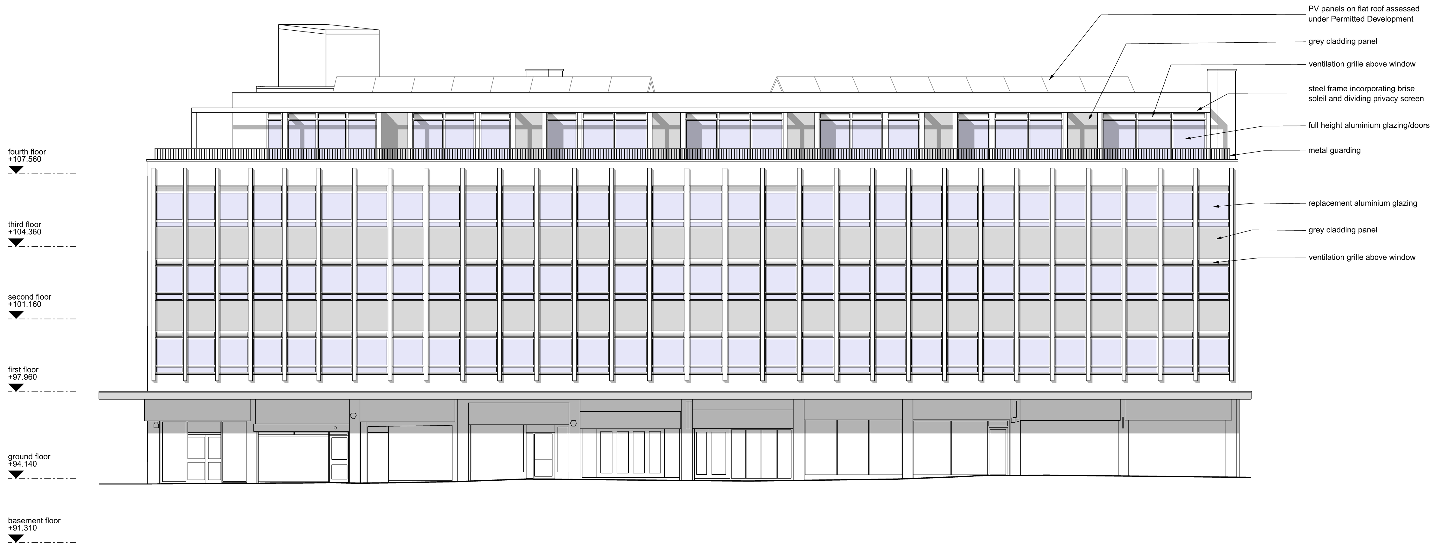
Elevation 02
