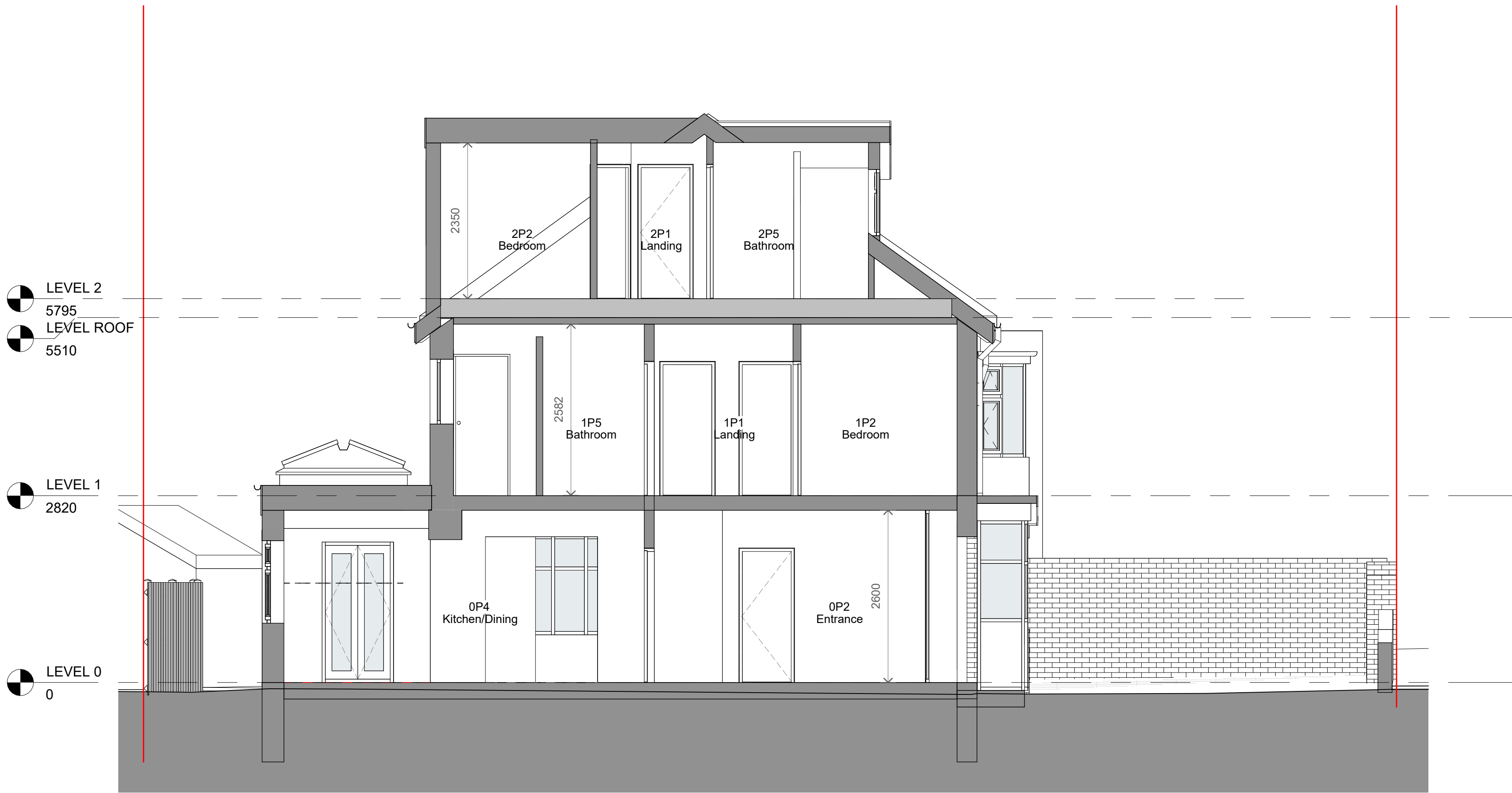
1 Section 9 1 : 50
