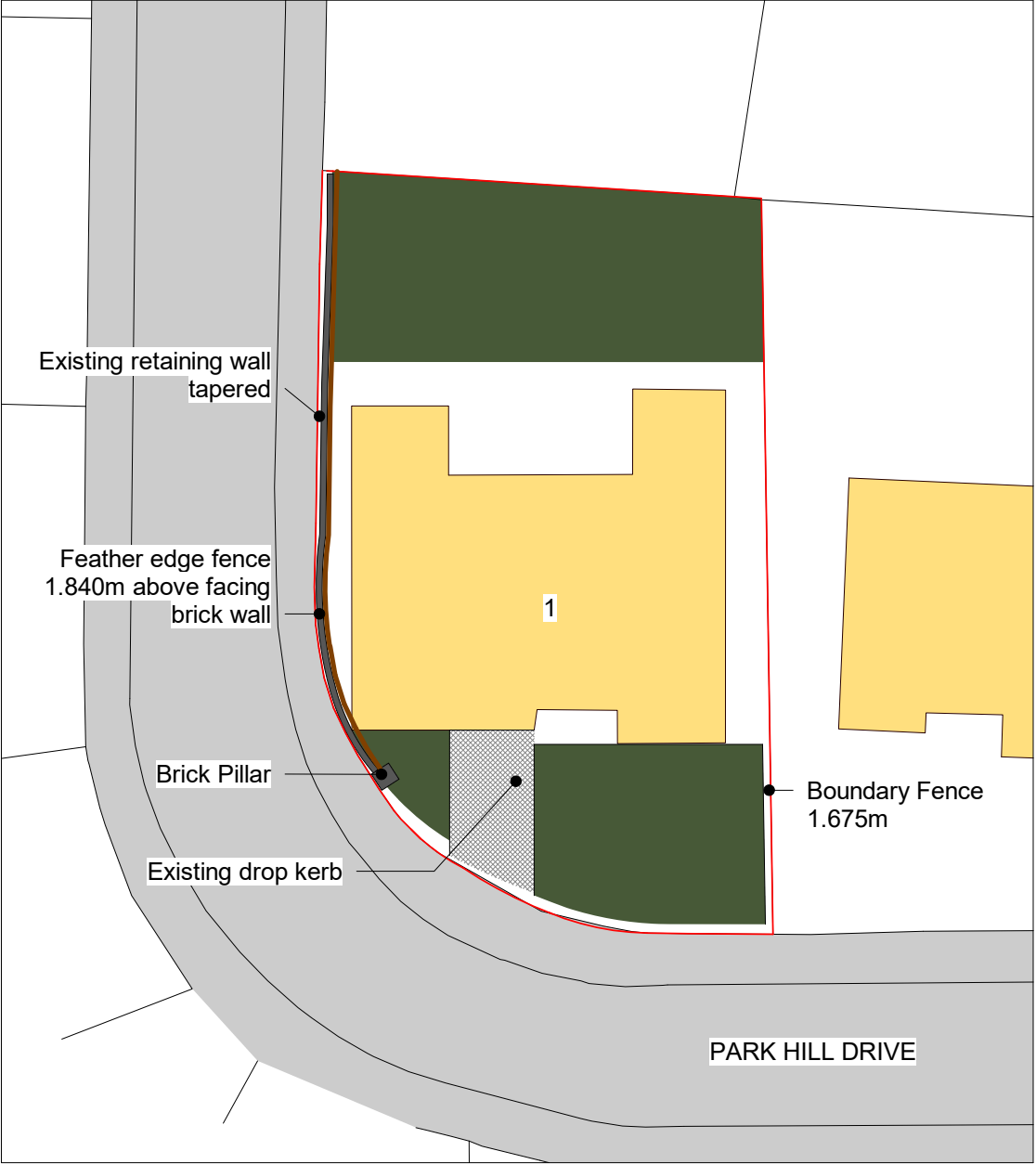
1. Site Existing 1 : 250
