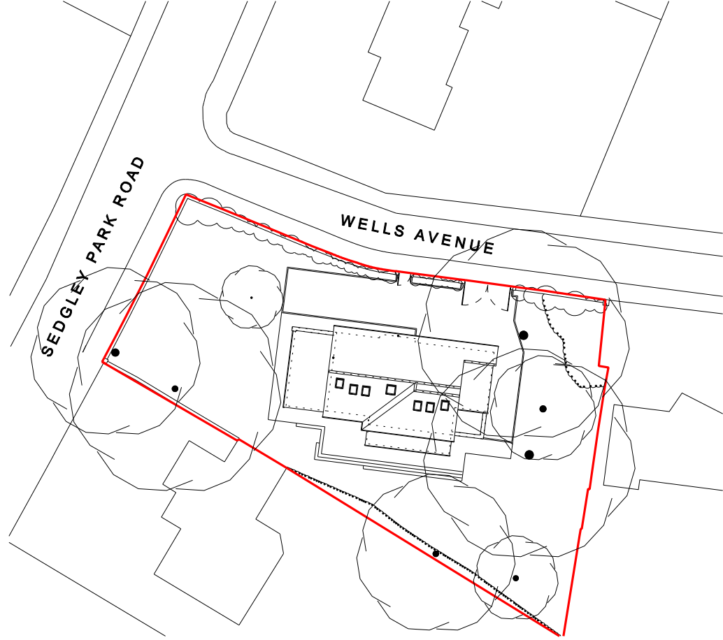
site plan 1:500
