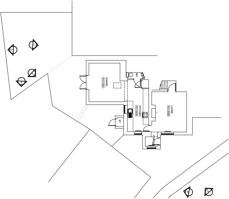
SITE PLAN 1:200
