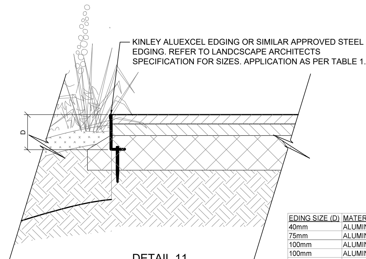
DETAIL 11 STEEL EDGE (SCALE 1:10)
