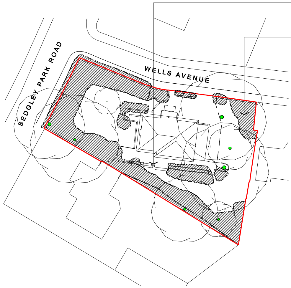
site plan, existing 1:500
