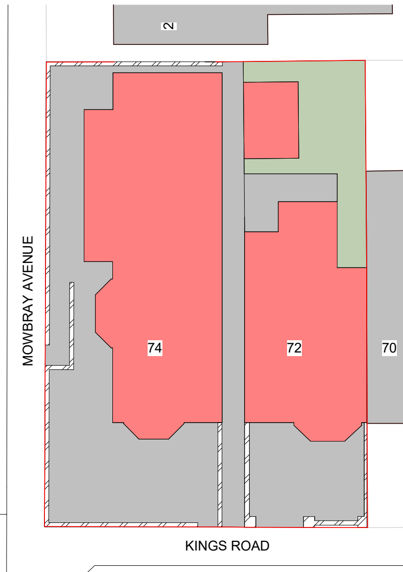
1 Site - Existing 1 : 200
