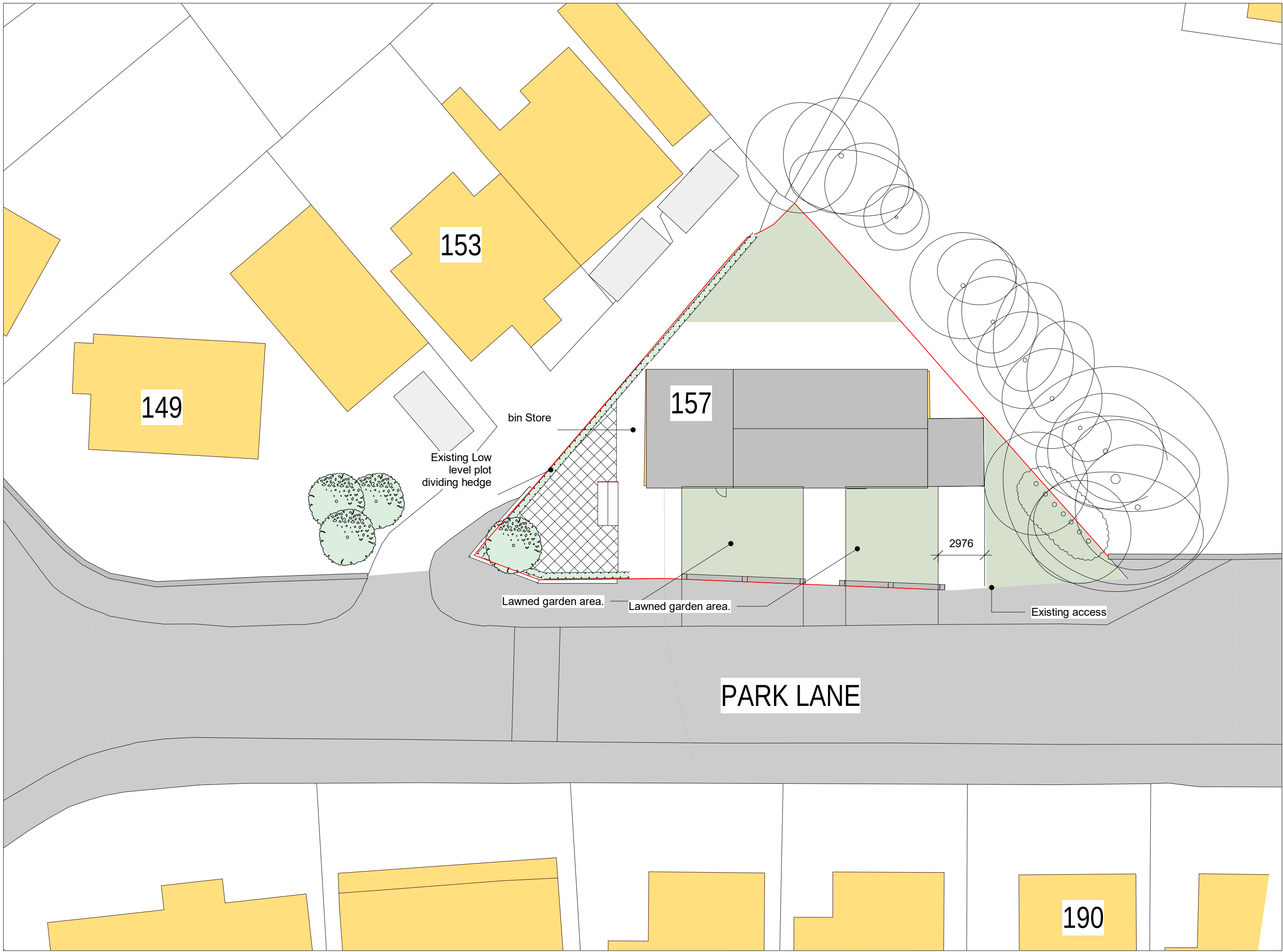
1 Site - Existing Site Layout Plan 1 : 200
