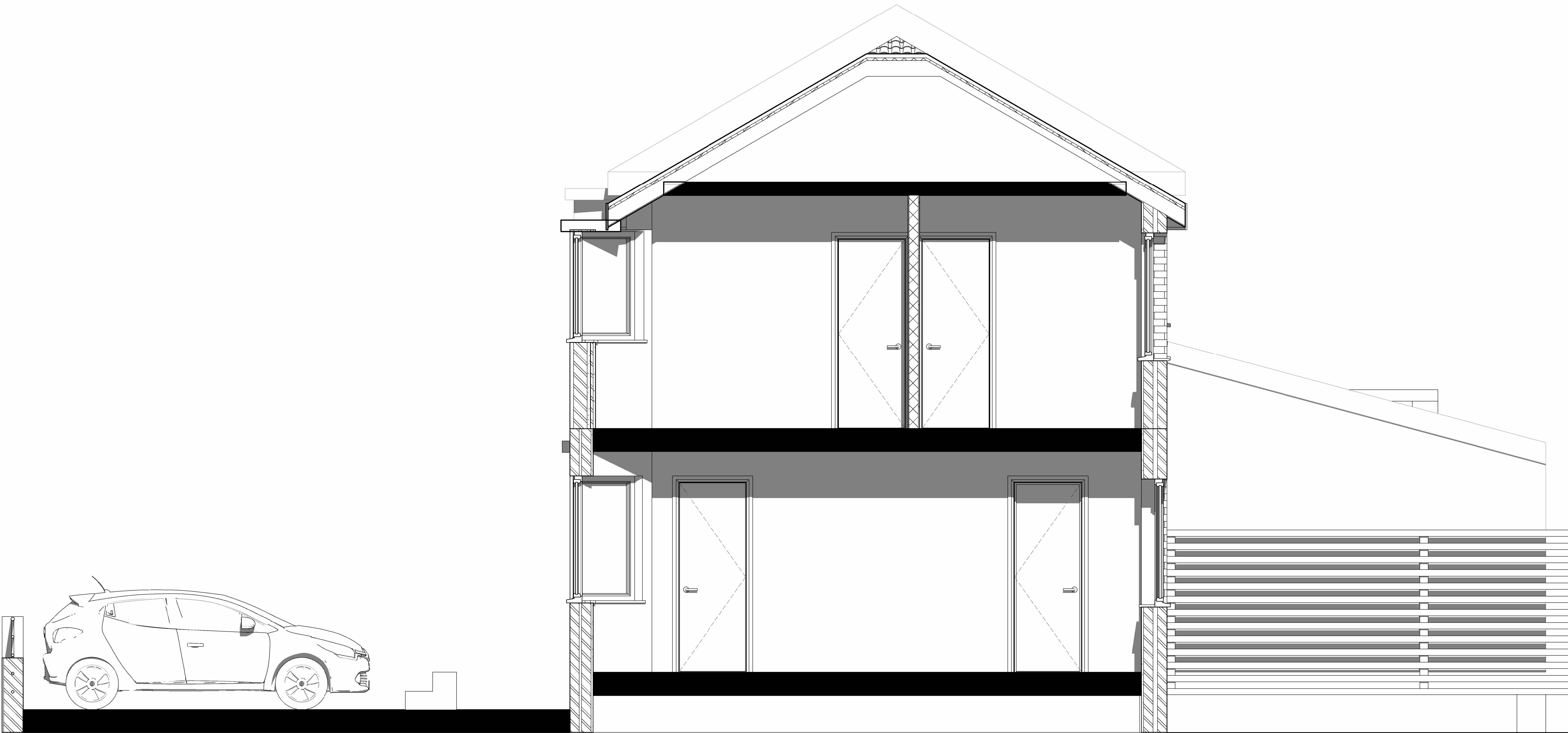
2 Existing - Section 2 1 : 25
