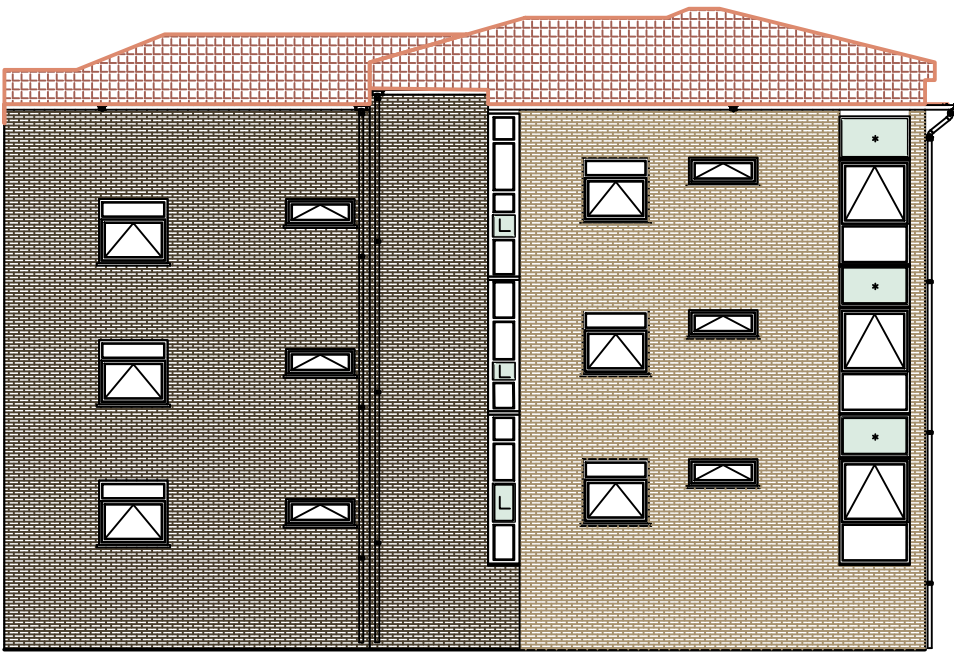
Elevation MP4
