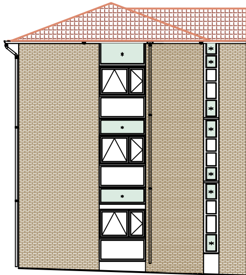
Elevation MP5
