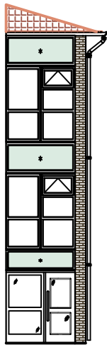
Elevation MP4
