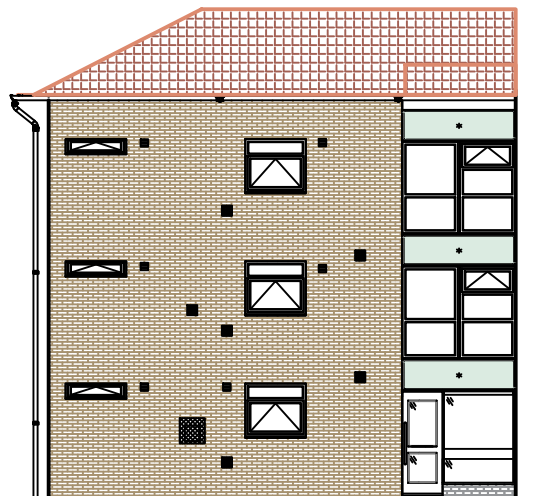
Elevation G
