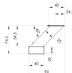
Pochwyt P4 inox dostępne długości: 580mm, 1000mm, 1500mm
