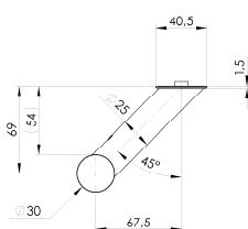
Pochwyt P2 inox dostępne długości: 580mm, 1000mm, 1500mm
