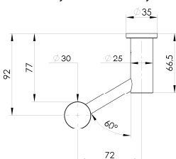
Pochwyt P1 inox dostępne długości: 580mm, 1000mm, 1500mm
