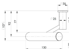
Pochwyt P3 inox dostępne długości: 580mm
