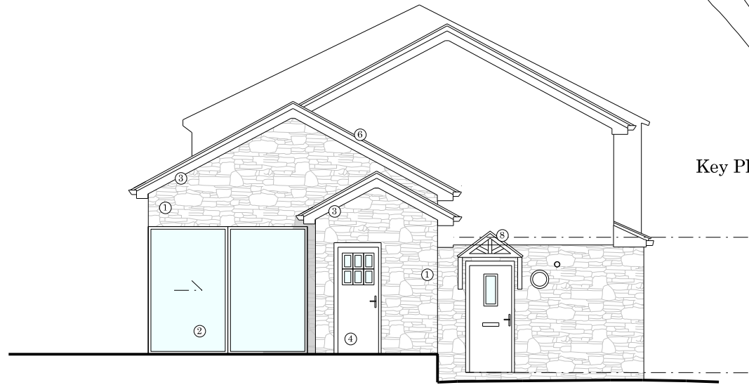
Elevation B
