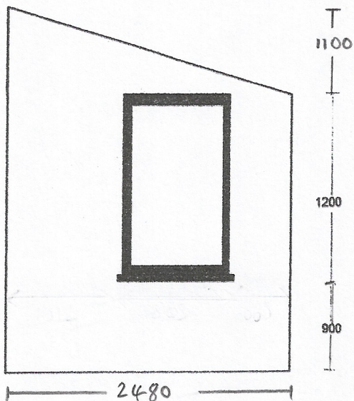
ELEVATION A
