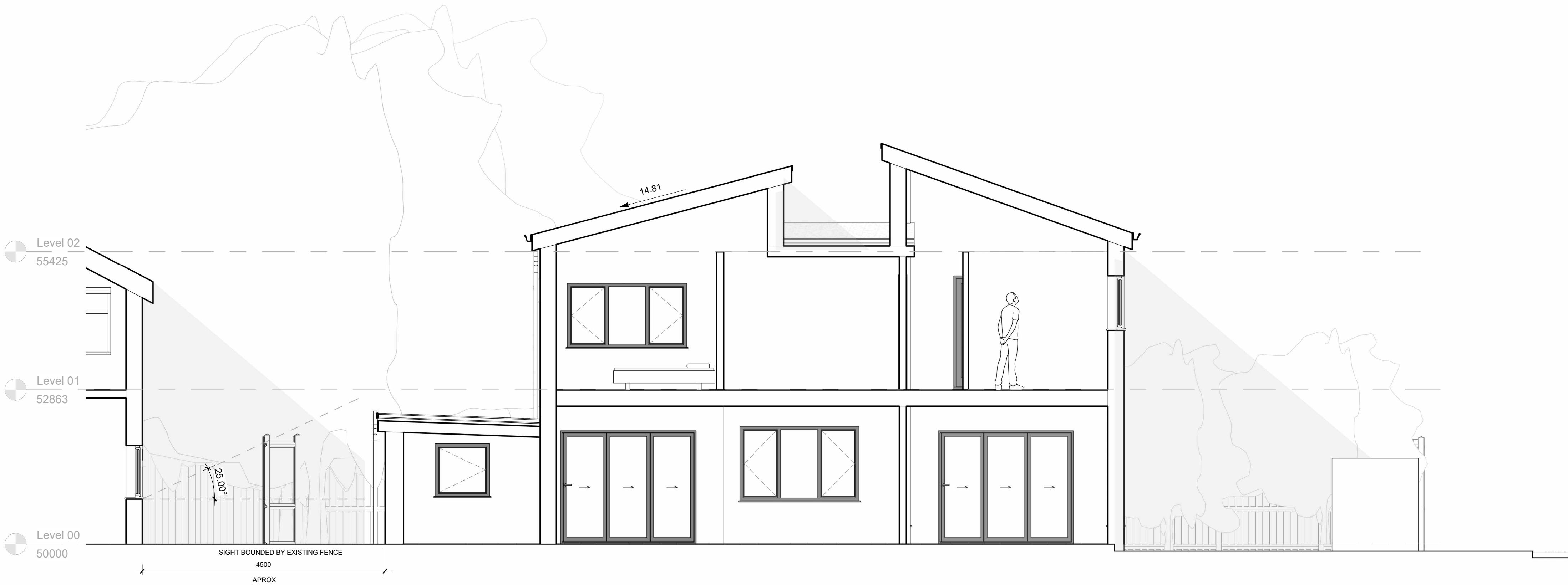
1 Site section Existing 1 : 50
