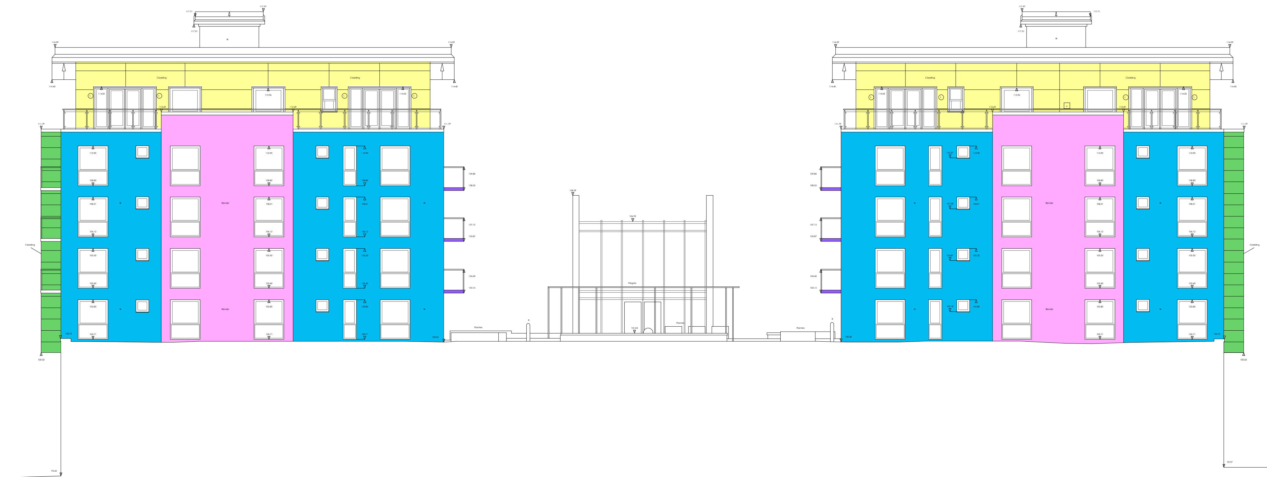
ELEVATION 6
