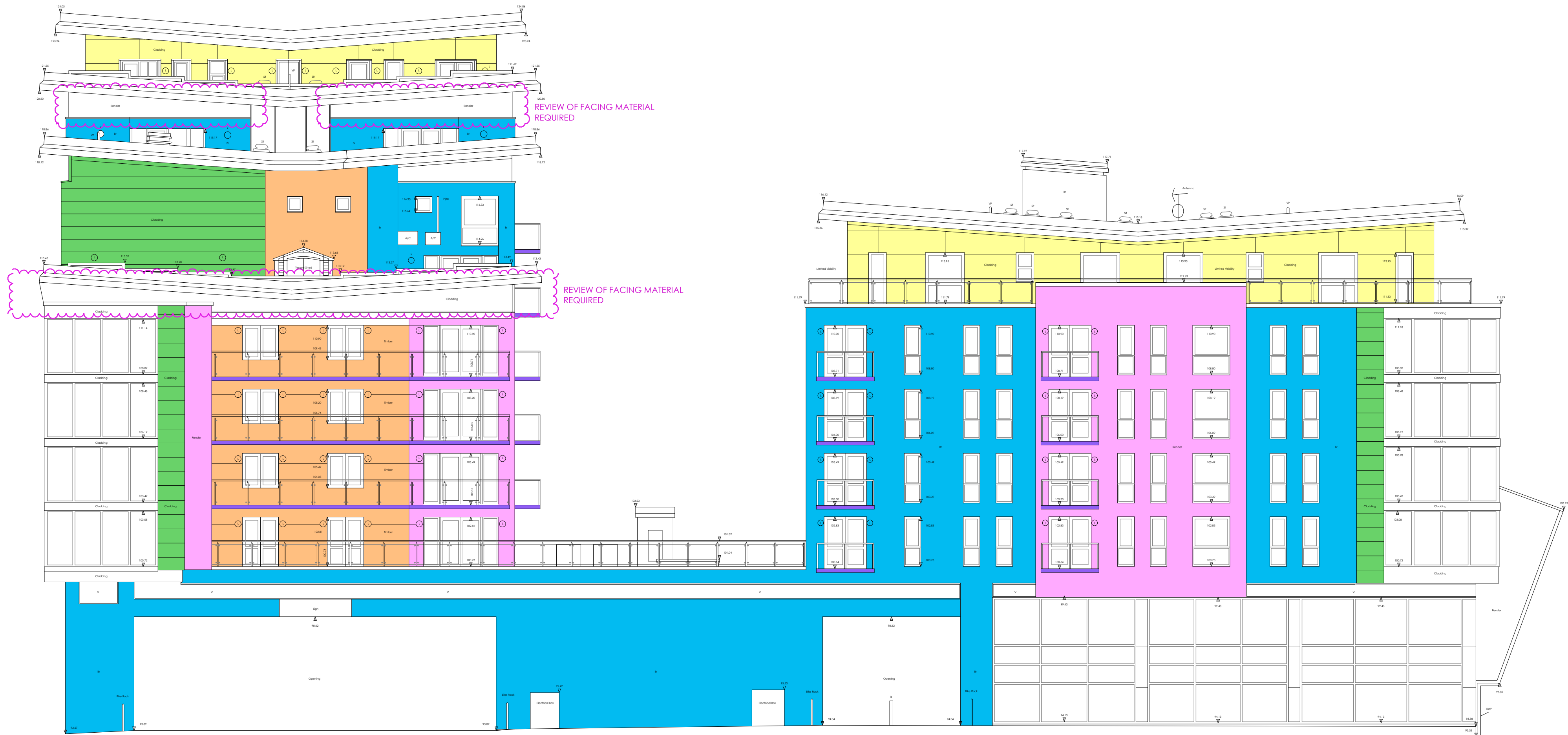
ELEVATION 1
