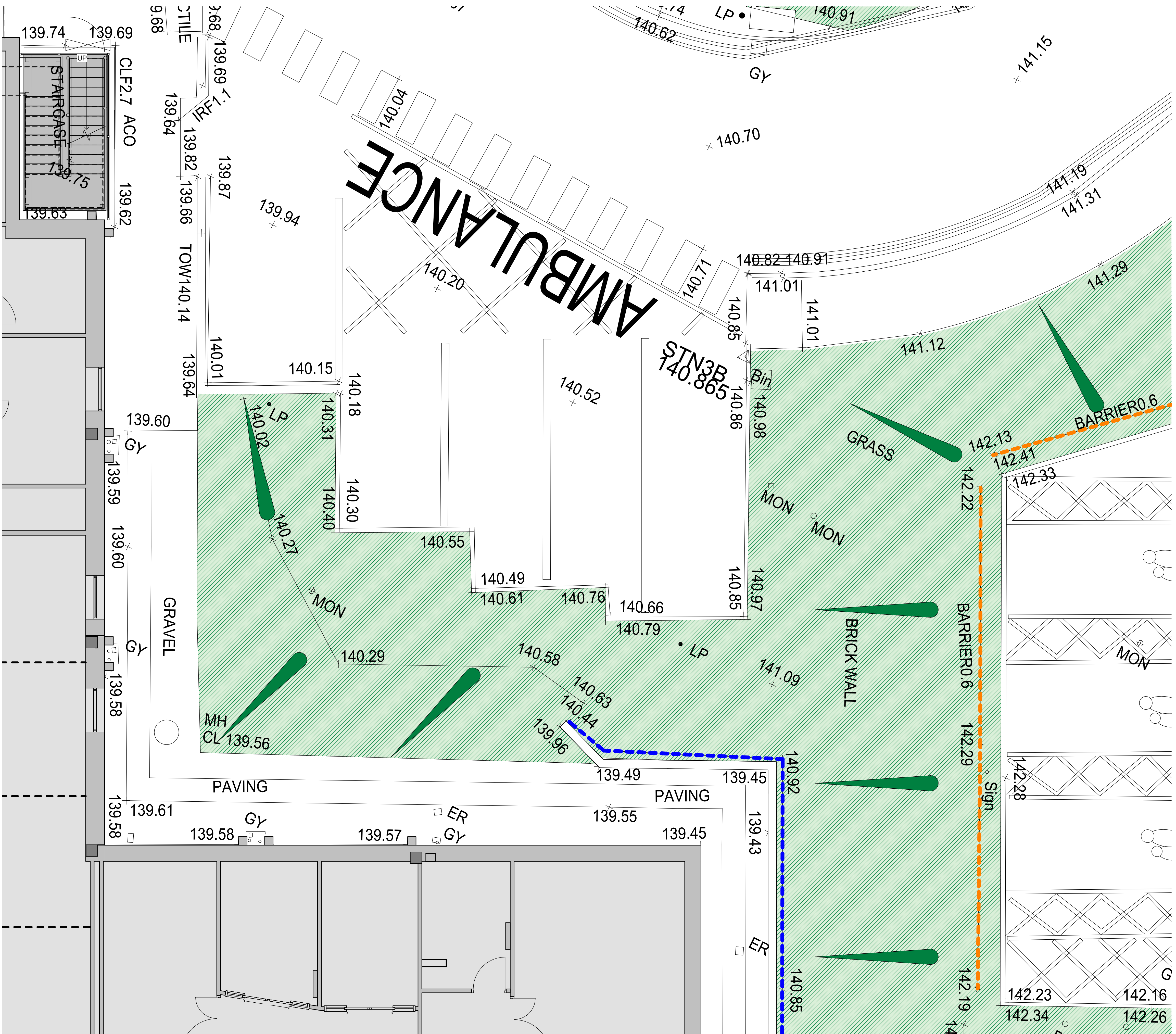
1 Existing GA Plan 1 : 50
