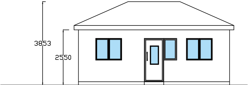
Elevation A
