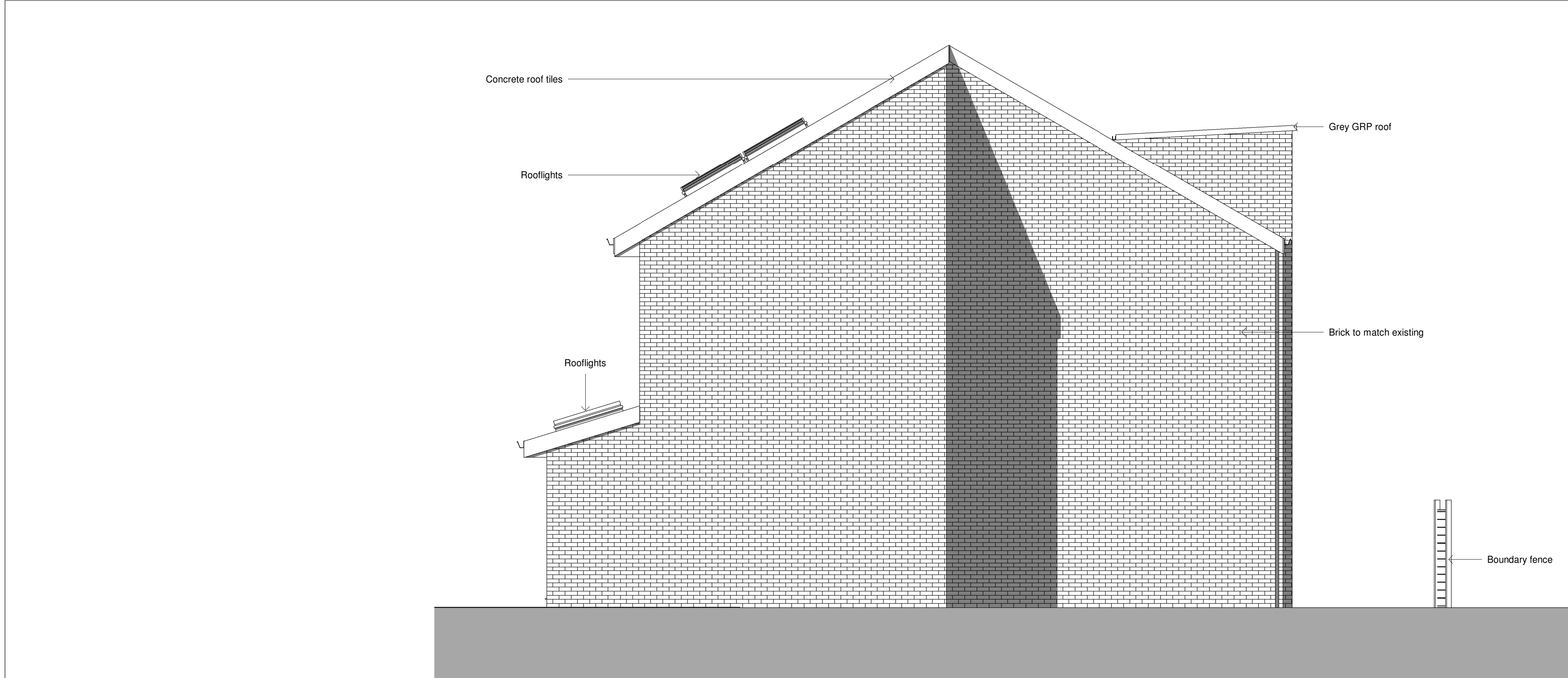
Side Elevation 01 1 : 50
