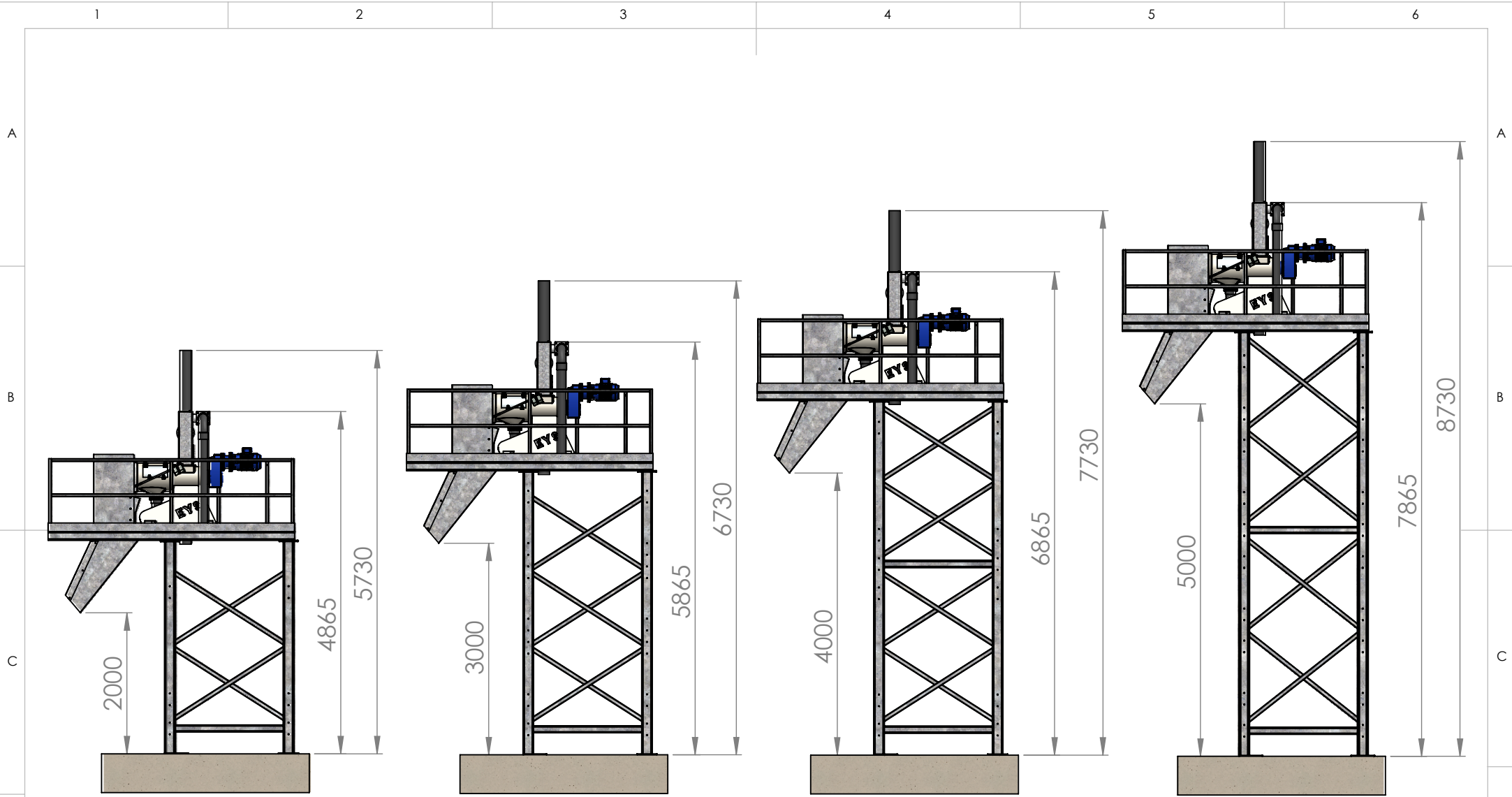
3m Overhung Gantry
