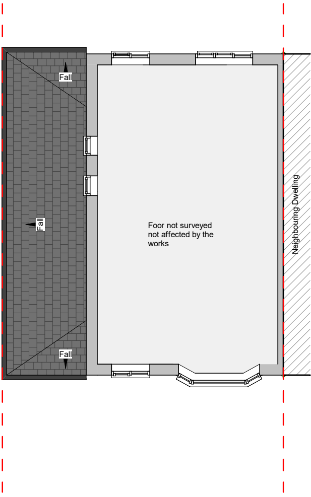
2 | Level 01_Existing 1 : 100
