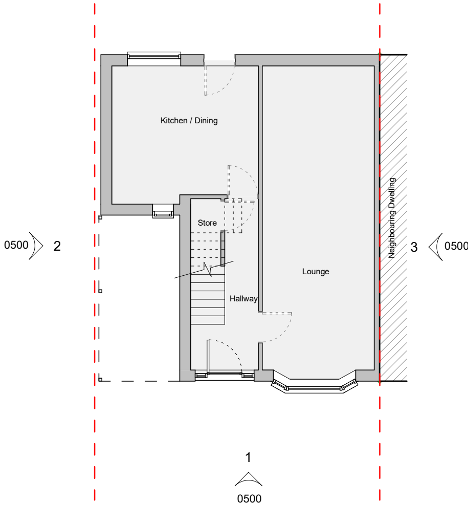
1 | Level 00_Existing 1 : 100
