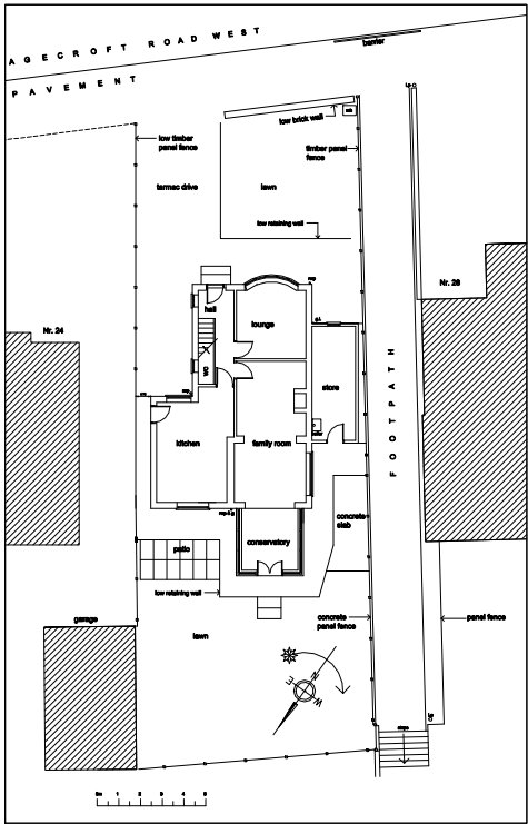
Site plan 1:200
